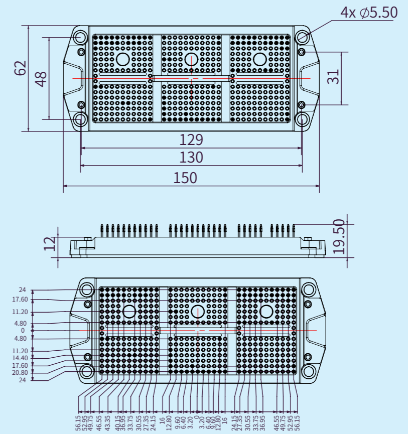
外型尺寸图 Outline Dimension
